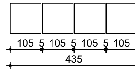
Blokpenanten voorgevel verdeling Hoogtemaatvoering gelijkverdelen
