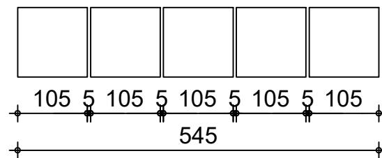
Blokpenanten achtergevel verdeling Hoogtemaatvoering gelijkverdelen
